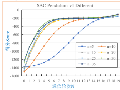
(b) 在 Pendulum-v1 中关于情形 S2 的得分
