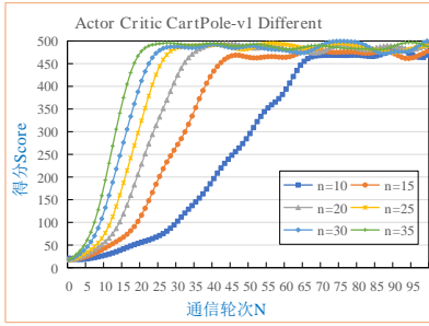
(d) 在 CartPole-v1 中关于情形 S2 的得分 图 5 搭载 Actor Critic 智能体的 GenFedRL 的得分
