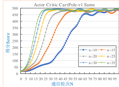
(b) 在 CartPole-v1 中关于情形 S1 的得分
