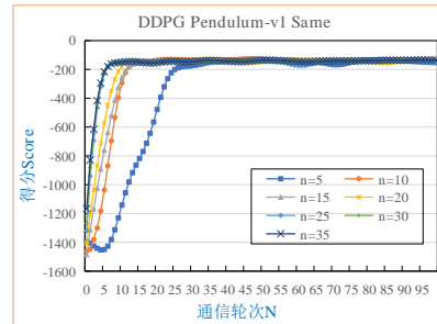
(a) 在 Pendulum-v1 中关于情形 S1 的得分
