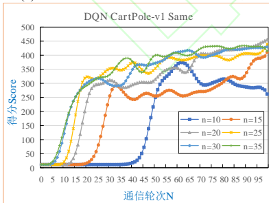
(b) 在 CartPole-v1 中关于情形 S1 的得分
