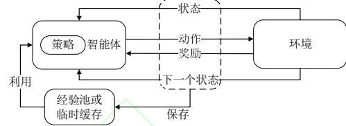
图 1 搭载异策略/同策略深度强化学习算法智能体的工作原理
