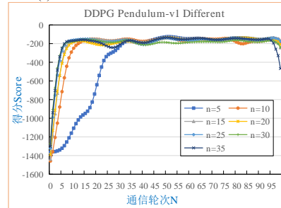
(b) 在 Pendulum-v1 中关于情形 S2 的得分
