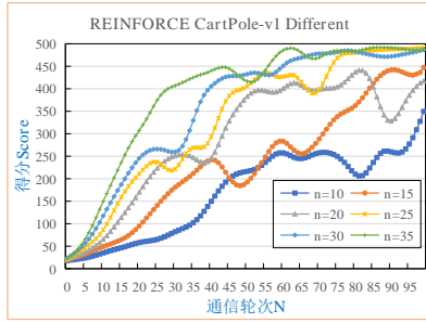
(d) 在 CartPole-v1 中关于情形 S2 的得分 图 3 搭载 REINFORCE 智能体的 GenFedRL 的得分
