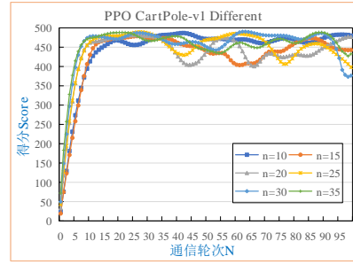
(d) 在 CartPole-v1 中关于情形 S2 的得分
