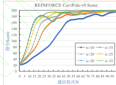
(a) 在 CartPole-v0 中关于情形 S1 的得分
