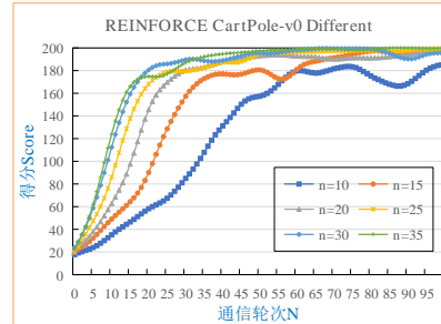
(c) 在 CartPole-v0 中关于情形 S2 的得分
