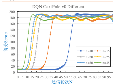
(c) 在 CartPole-v0 中关于情形 S2 的得分
