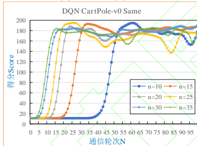
(a) 在 CartPole-v0 中关于情形 S1 的得分
