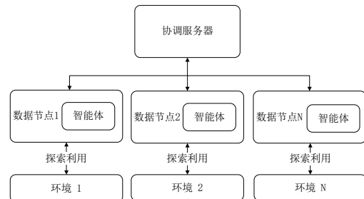
图 2 通用联邦强化学习框架 GenFedRL
